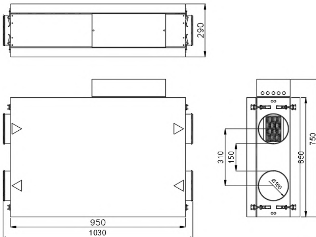
Zenit Standart 200 E
